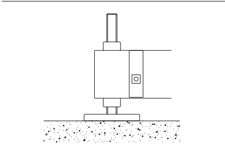
Quattro vitoni di livellamento Four levelling screw-jacks
