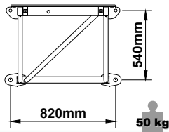
Dettagli modulo ponte Deck module details
